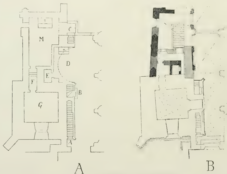
Fig. 32. Dwa plany wieży północnej i przyległych kaplic.
